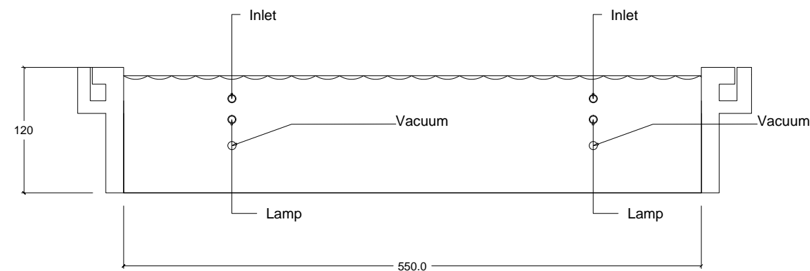
Elevation B
